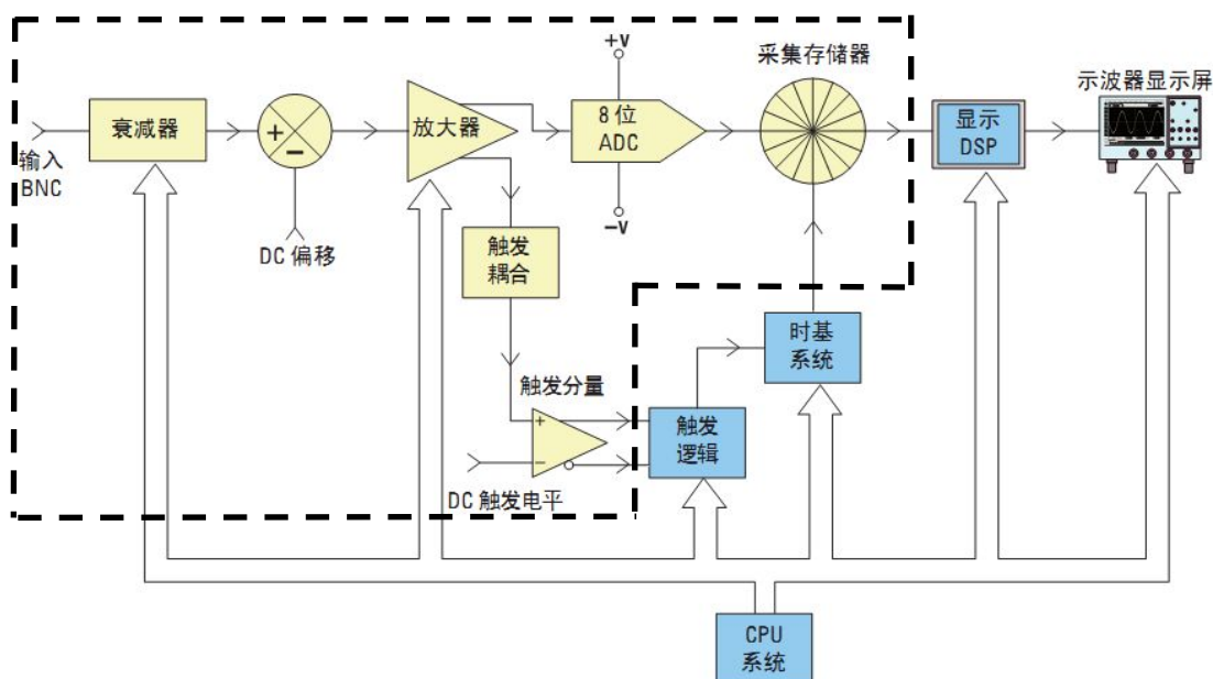
图 1: 数字存储示波器 (DSO) 一个通道信号处理过程的模块化示意图。其中虚线框内的组件是一个信号通道专用的 (多通道示波器就有多套这样的组件); 框外组件表示所有信号通道共用的系统组件。CPU 和 DSP 分别是 Central Processing Unit(中央处理器)和 Digital Signal Processor (数字信号处理器) 的简称。(本示意图是在网络图片的基础上修改而成。)
