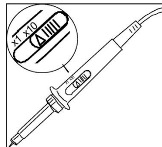
图 2: 输入导线上的 X10 衰减开关。
